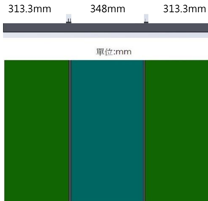
圖 02、部分競賽軌道尺寸示意圖
