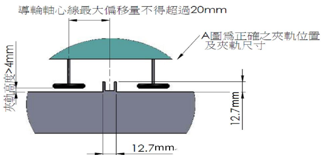
圖 2、軌道夾軌尺寸示意圖
